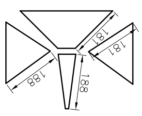
RUDDER POD
